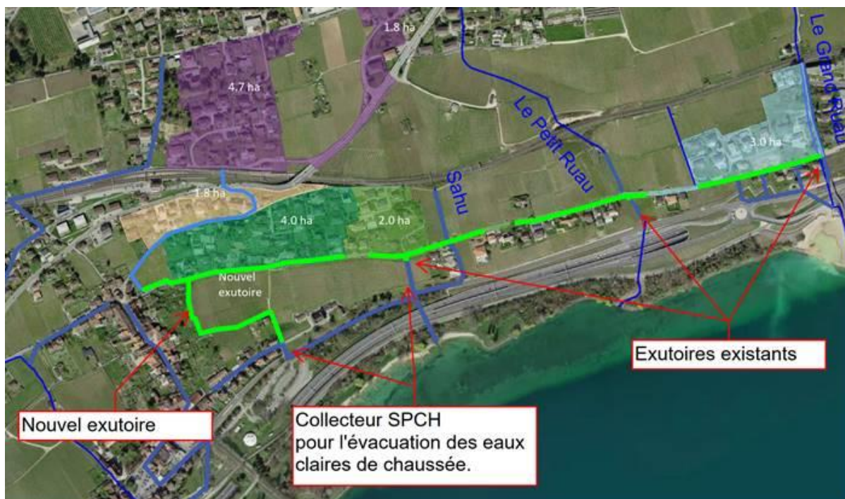
Schéma complet du futur réseau d'évacuation d'eaux claires de la route des Clos.
